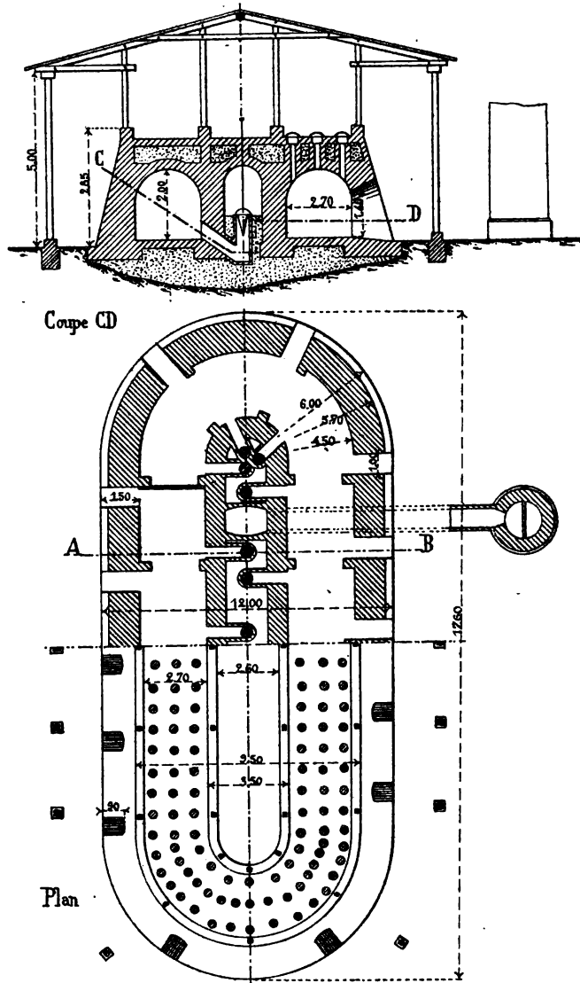
Fig. 72, 73. — Four Hoffmann ovale à 14 compartiments.
